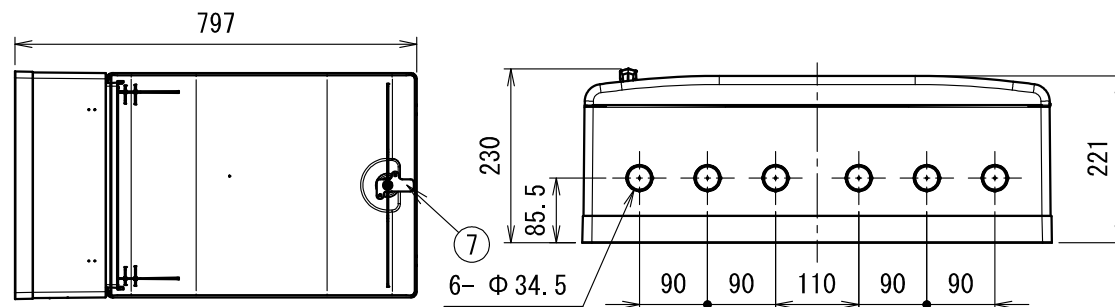
蓋全開時参考図 (1/15)
